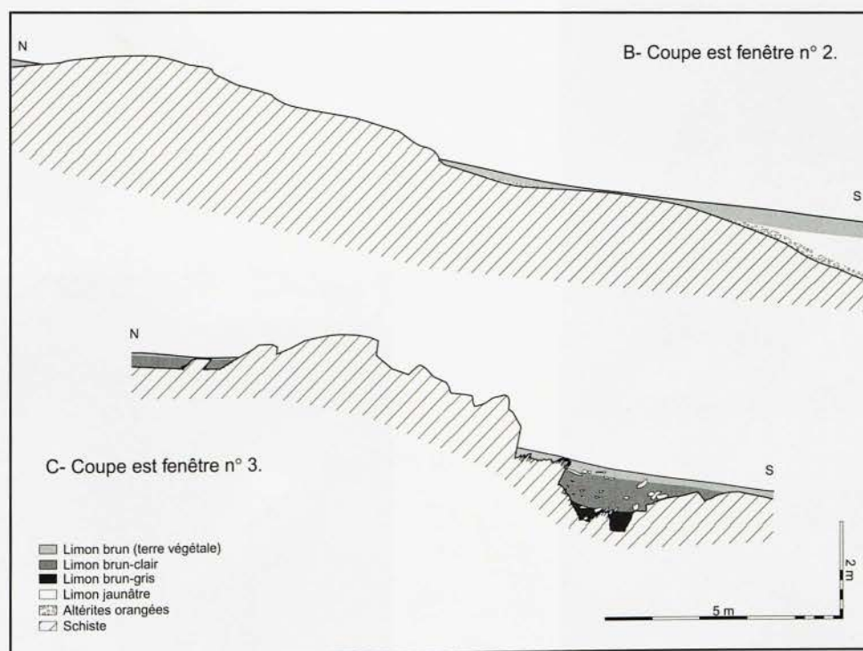
Fig. 52 - SAINT-GERMAIN-DU-CORBÉIS, l'Ermitage. Organisation de la carrière (A), profil naturel (B), profil perturbé par un front de taille au niveau de l'affleurement principal du schiste (C).
