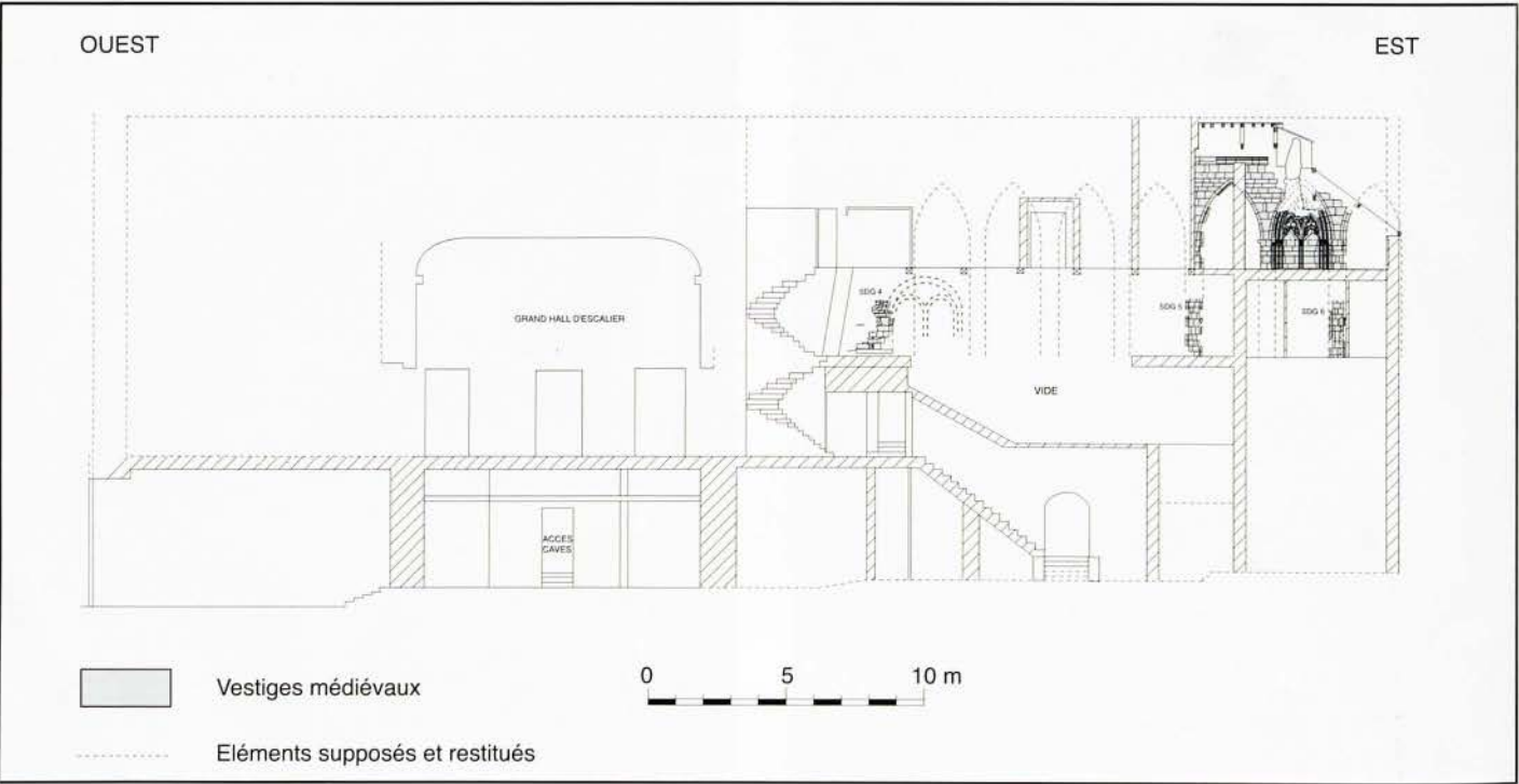
Fig. 16 - LISIEUX, ancien palais épiscopal. Elévation du parement sud du mur longitudinal de refend.
