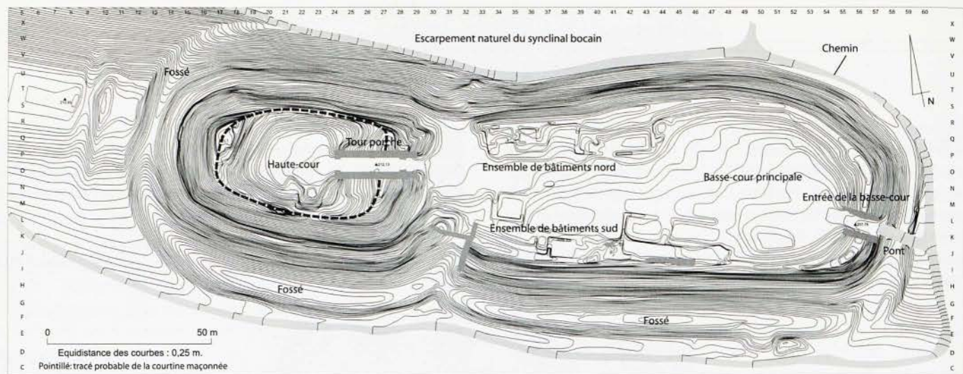
Fig. 13 - LA POMMERAYE, Château Ganne. Relevé altimétrique de l'ensemble castral.
