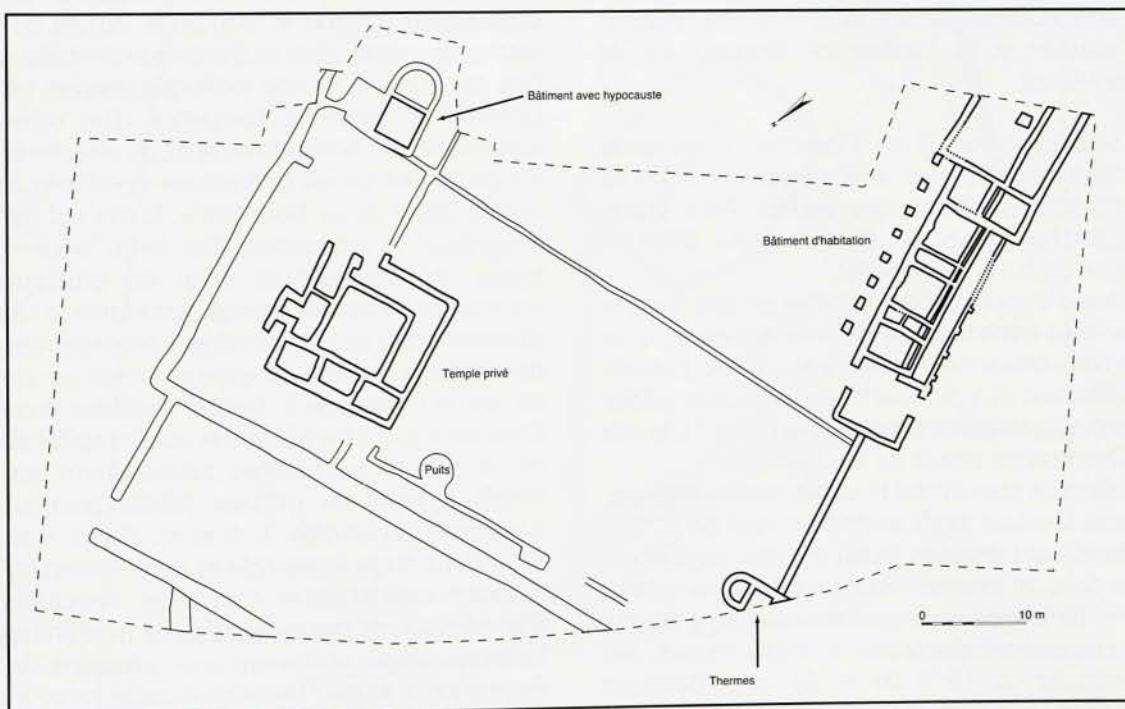
Fig. 42 - MARCEI, la Chasnière. Relevé en plan de la villa du Bas-Empire.
