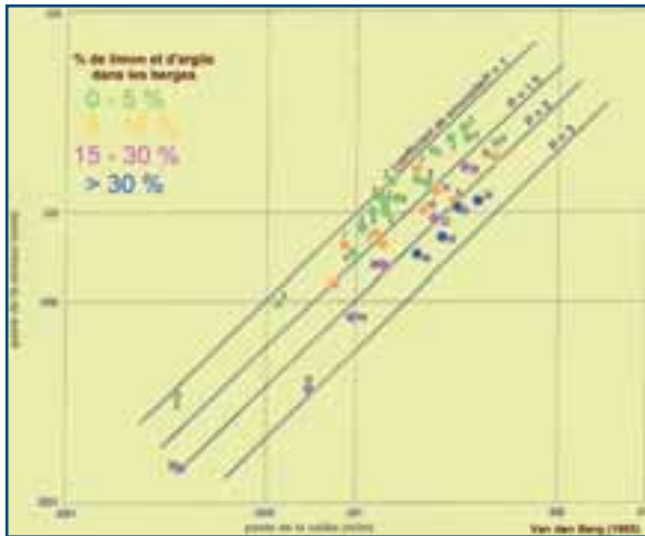
↑ Figure 89 : Relation entre le coefficient de sinuosité (ici mesuré par le rapport pente de la vallée/pente du lit) et la nature des berges. Noter que les cours d'eau sinueux à très sinueux sont caractérisés par des berges non cohésives. Les cours d'eau très méandriques ( P > 2 ) ont eux des berges plutôt très cohésives (d'après Van den Berg, 1995). ≈
