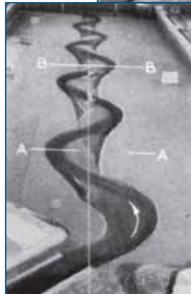
↑ Figure 90 : Exemple de tracé en plan très homogène tel que l'on en obtient en laboratoire. Berges et fond sableux : en haut, conditions initiales, en bas, après 3 h d'écoulement (Friedkin, 1945). ≈
