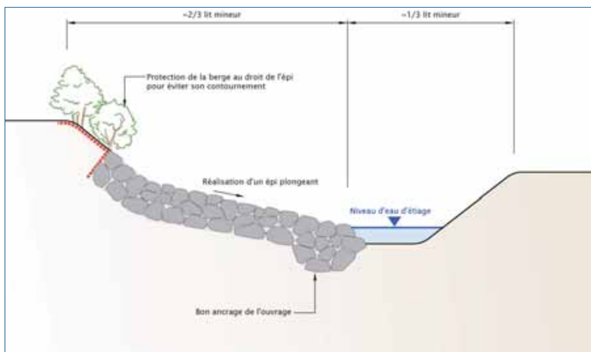
↑ Figure 9 : Schéma « type » d'un épi plongeant en blocs (figure Biotec). 🌊
