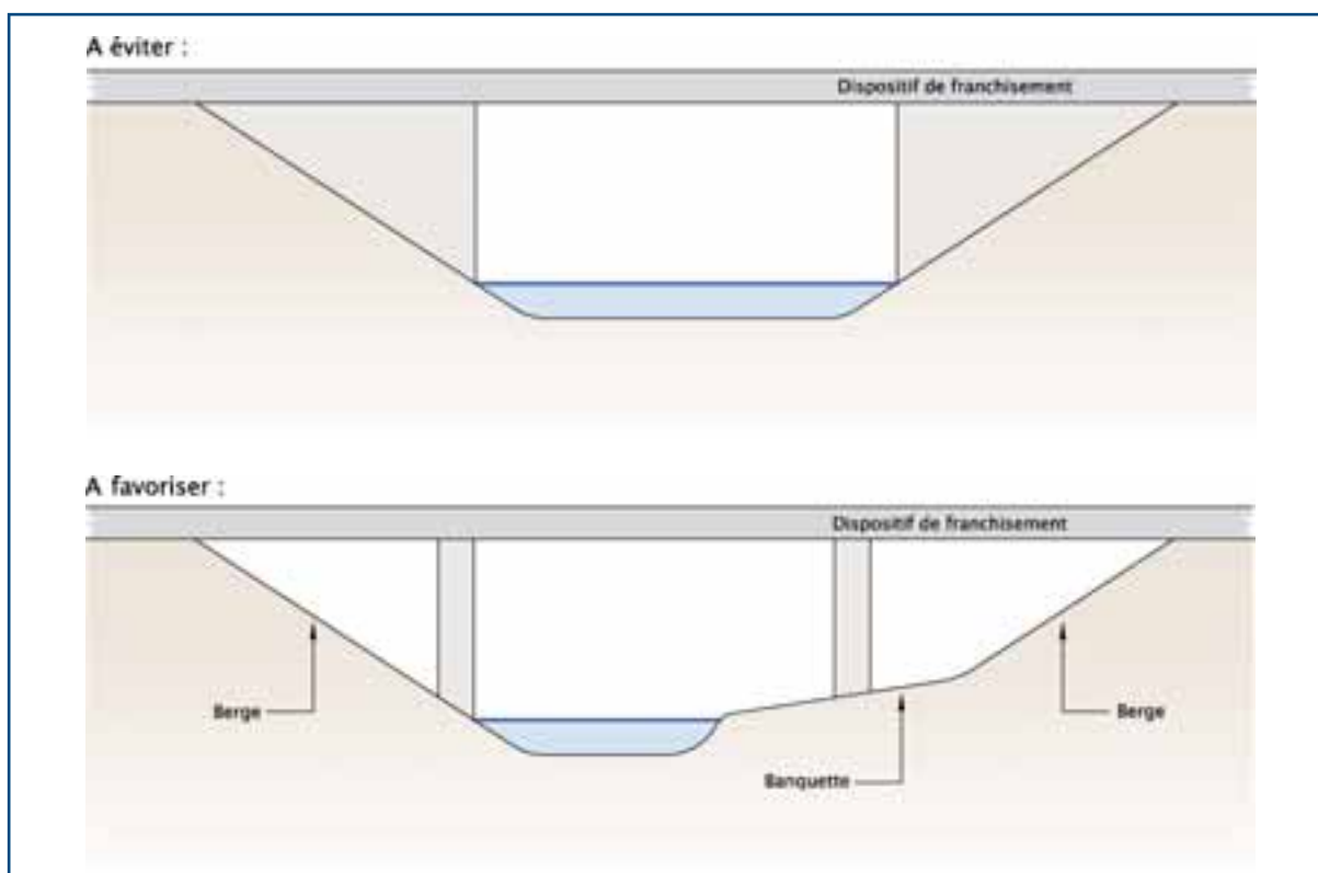
↑ Figure 104 : Exemple de configuration de franchissement à éviter en haut et à favoriser en bas. ≈
