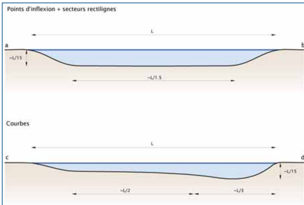
↑ Figure 95 : Exemple de profils en travers (voir le paragraphe précédant pour l'implantation des profils). ≈
