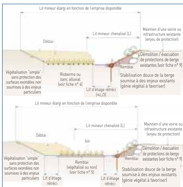
Figure 61 : En haut, exemple d'un profil type de restauration d'un cours d'eau anciennement chenalisé élargi avec la suppression d'anciennes protections de berges et la réalisation de risbermes et d'un lit d'étiage rétréci. En bas, idem avec la création d'un îlot central (figure Biotec). ≈
