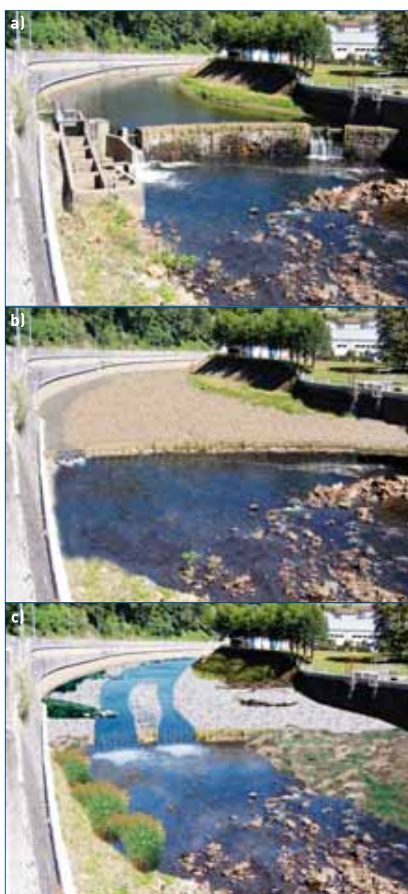
Figure 40 : Exemple d'un photomontage illustrant un seuil sur la Corrèze à Tulle dans son état initial, en cours de démolition et une fois le site réaménagé en fin de travaux (source : Malavoi, Biotec, 2005).
