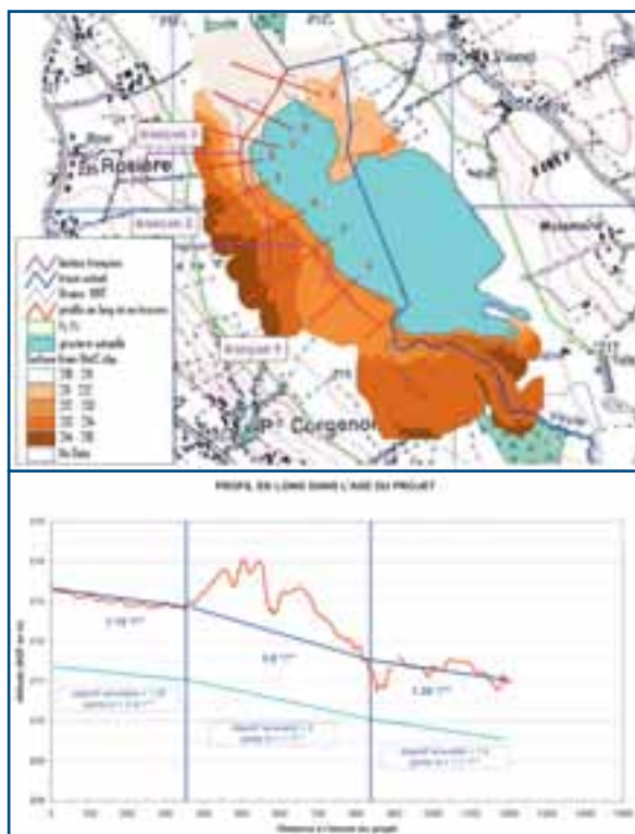
Figure 85 : Projet de dérivation de la Veyre au droit de la gravière de St-Denis-les-Bourg. Etude fine de la topographie avec en haut un plan de situation et en bas le profil en long du tracé le plus favorable (étude Biotec-Malavoï, 2005). ≡
