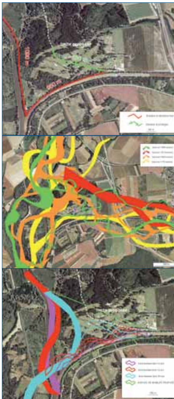
Figure 49 : Exemple d'analyse prédictive du tracé de deux cours d'eau à leur confluence suite à la suppression des contraintes latérales. En haut, contexte local des protections existantes et de leur report en arrière pour protéger un golf existant mais qui sera en partie déplacé. Au centre, analyse historique des tracés. En bas, simulation du tracé à 10 et 50 ans (source : Malavoi, 2005). ≈
