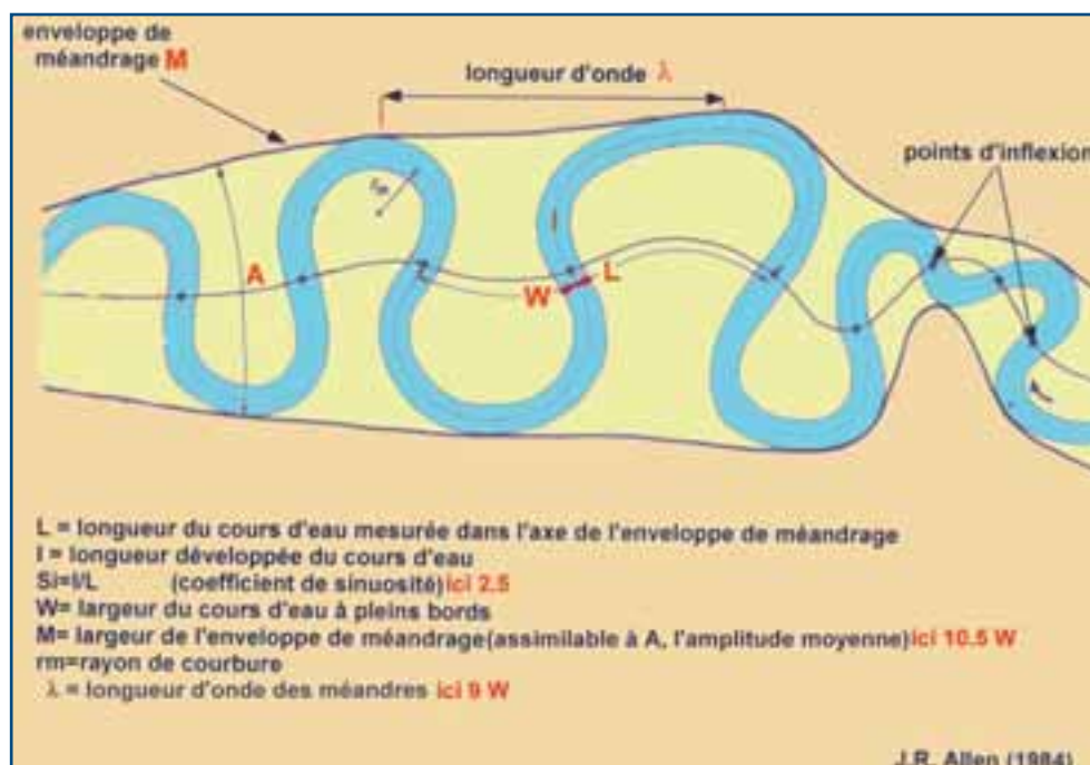
Figure 88 : Mesures morphométriques sur un cours d'eau sinueux. Nota : la largeur « à pleins bords » [sur cette figure « W »] d'un cours d'eau se mesure au droit des points d'inflexion où le profil en travers est le plus symétrique [d'après J.-R. Allen, 1984].
