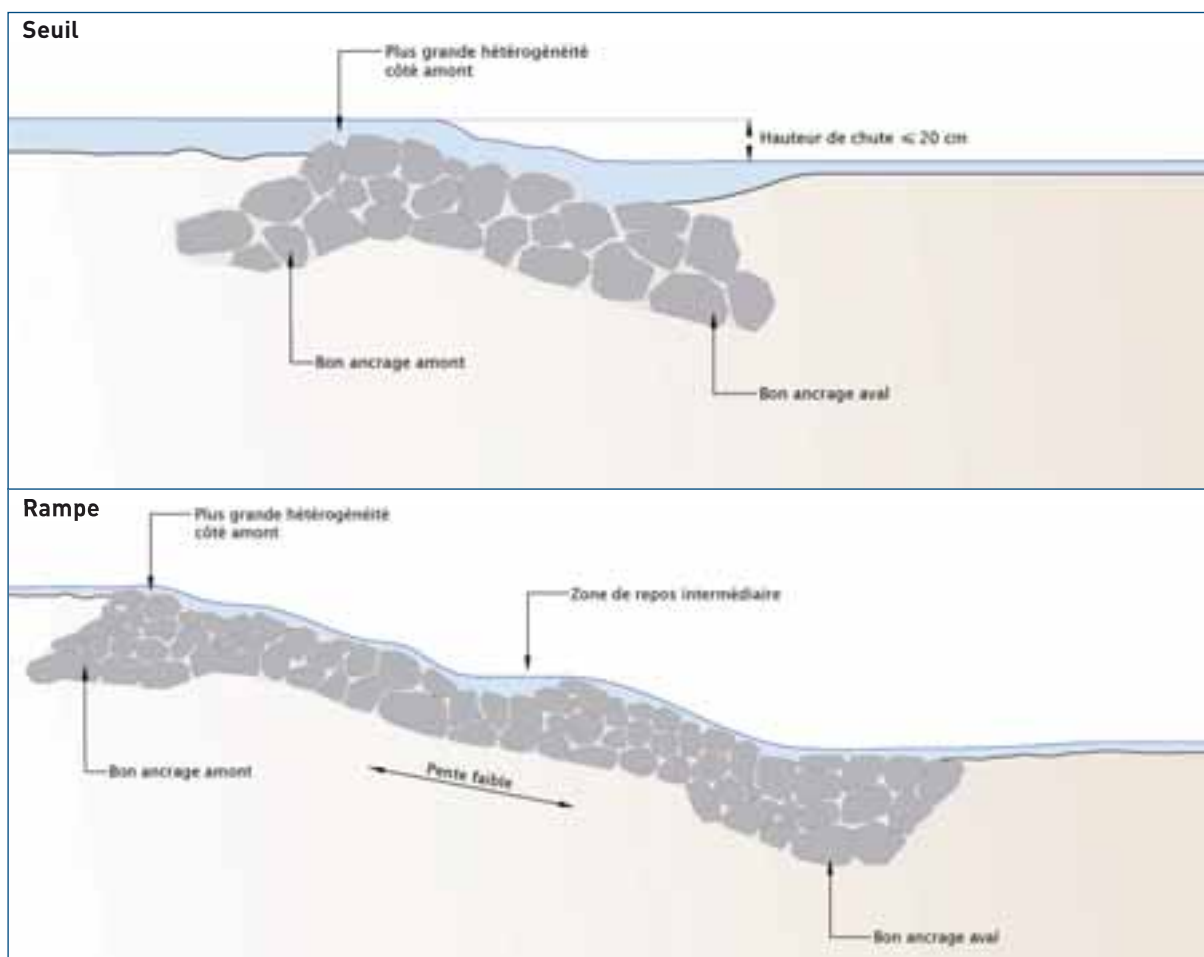
Figure 24 : Illustration de principes à respecter dans la réalisation de seuils (en haut) ou de rampes (en bas) pour garantir la franchissabilité piscicole. ≈
