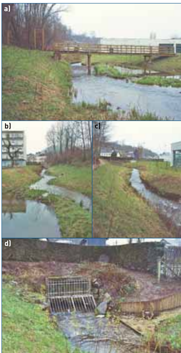
Figure 66 : Vues du site en date du 26.02.07. a) Tronçon médian avec un élargissement du lit mineur et la création d'un bras mort. b) Lit « méandri-forme » réalisé à l'amont de la passerelle. c) Lit restauré à l'aval de la passerelle. d) Détail de la grille à l'aval du tronçon restauré, où le Bolbec « replonge » dans sa canalisation. ≈
