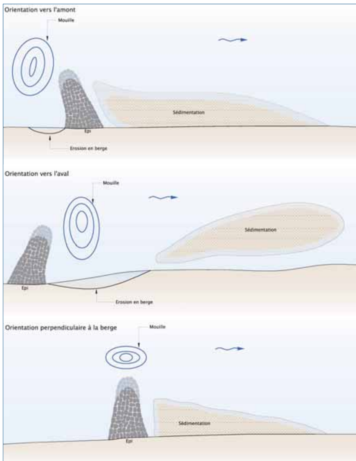
↑ Figure 8 : Illustration schématique de différents effets produits sur la diversification des substrats ou des hauteurs d'eau liées à l'orientation des épis (figure Biotec). ≡
