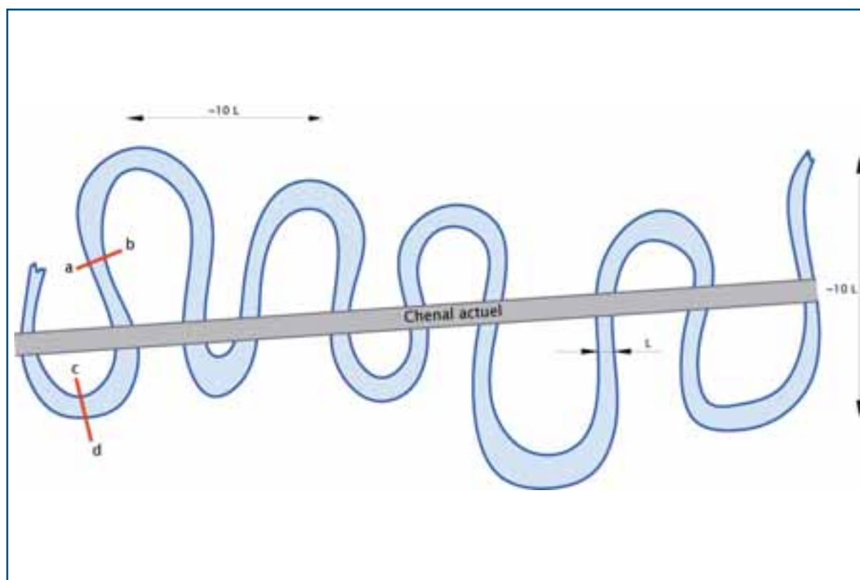
Figure 94 : Exemple de tracé en plan méandrique irrégulier (voir § suivant pour les profils types). ≈
