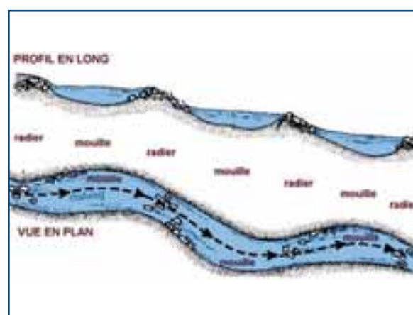
↑ Figure 92 : Forme typique du profil en long d'un cours d'eau sinueux. ≡
