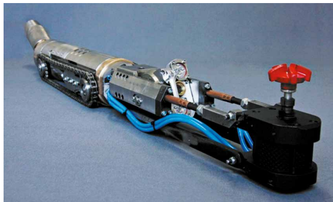
Robot fraiseur.
