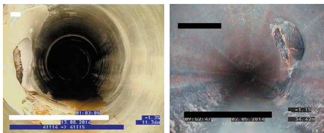
Réhabilitation d'un branchement avant/après.
